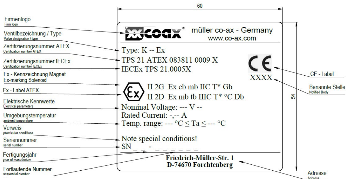
Abbildung 1.7.1 Typenschild Ex-Magnet mit Beispielbeschriftung
