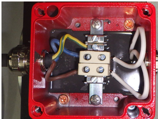
Abbildung 5.3.1: Anschlusskasten mit Klemmleisten
