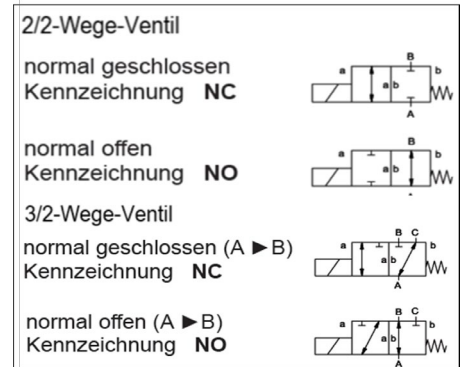
Abbildung 2.1.1 Schaltbilder Ventile
