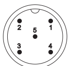
Stecker Lötseite
